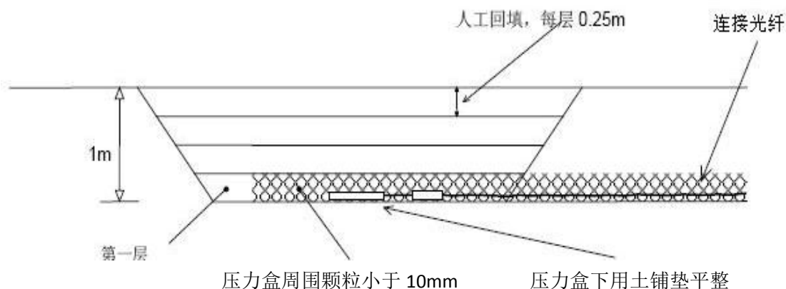
图 3.3.1 光纤光栅土压力计安装示意图（一）
